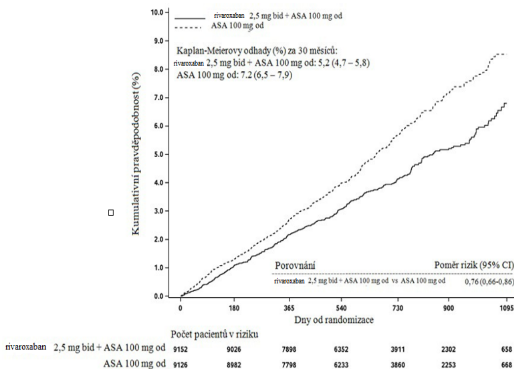
Obrázek 2: Čas do prvního výskytu primárního parametru účinnosti (cévní mozková příhoda, infarkt myokardu, kardiovaskulární úmrtí) ve studii COMPASS
